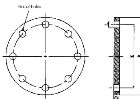
TYPE 05 : BLANK FLANGE
